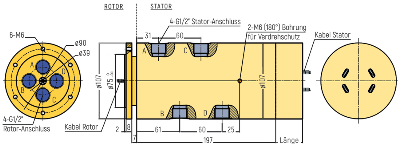
RX-PN1204-QS2-B - G1/2" Anschluss
