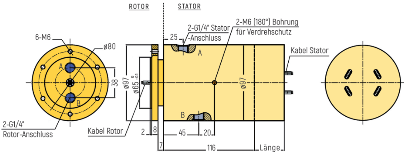
RX-PN1402-QS2-B - G1/4" Anschluss
