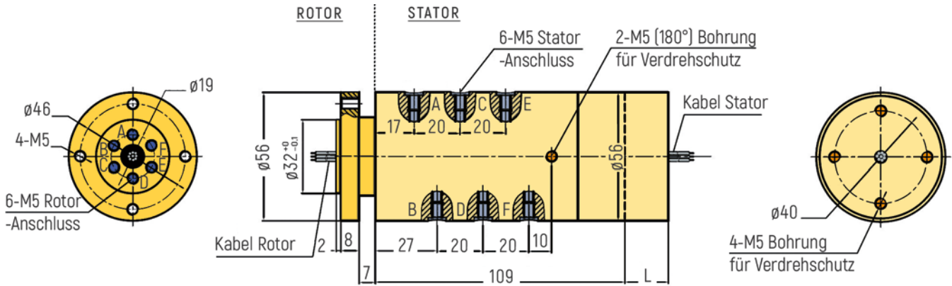
RX-PNM506-QS1-B - M5 Anschluss
