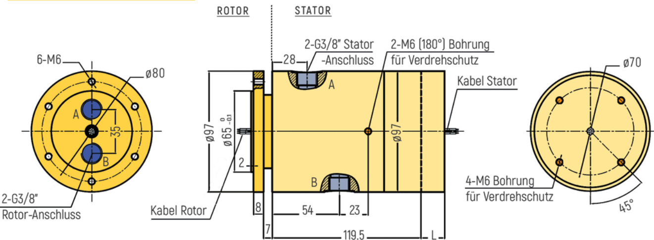
RX-PN3802-QS1-B - G3/8" Anschluss
