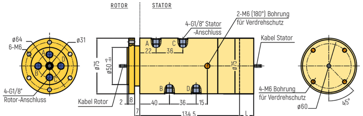
RX-PN1804-QS1-B - G1/8" Anschluss
