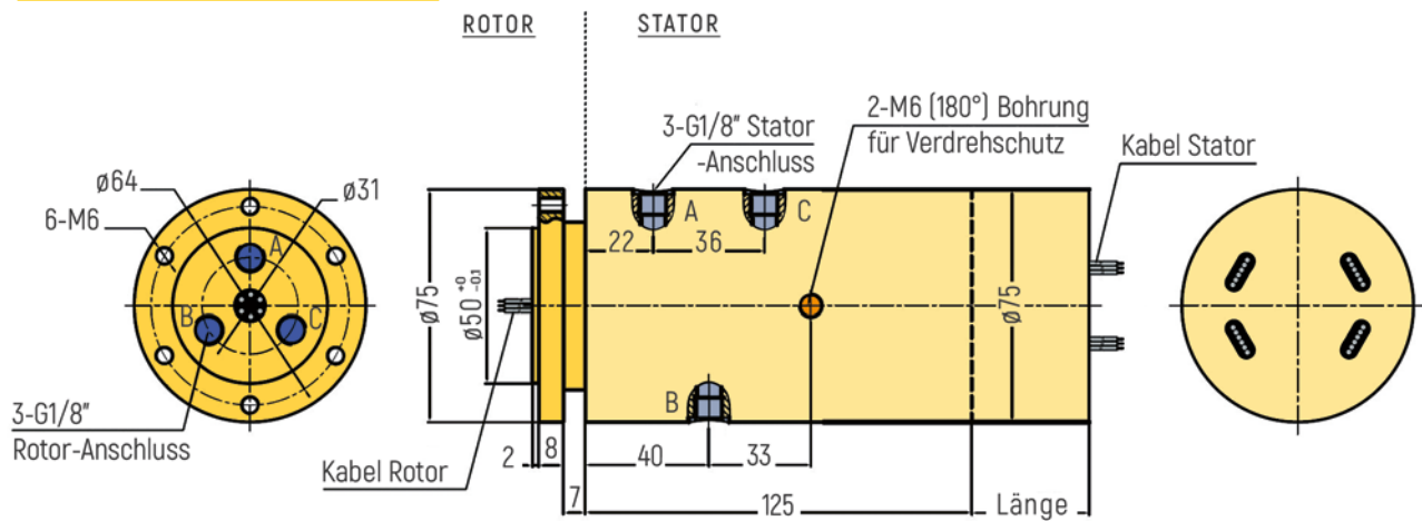
RX-PN1803-QS2-B - G1/8" Anschluss
