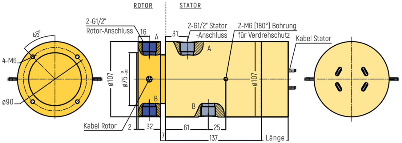
RX-PN1202-QS2-C - G1/2" Anschluss
