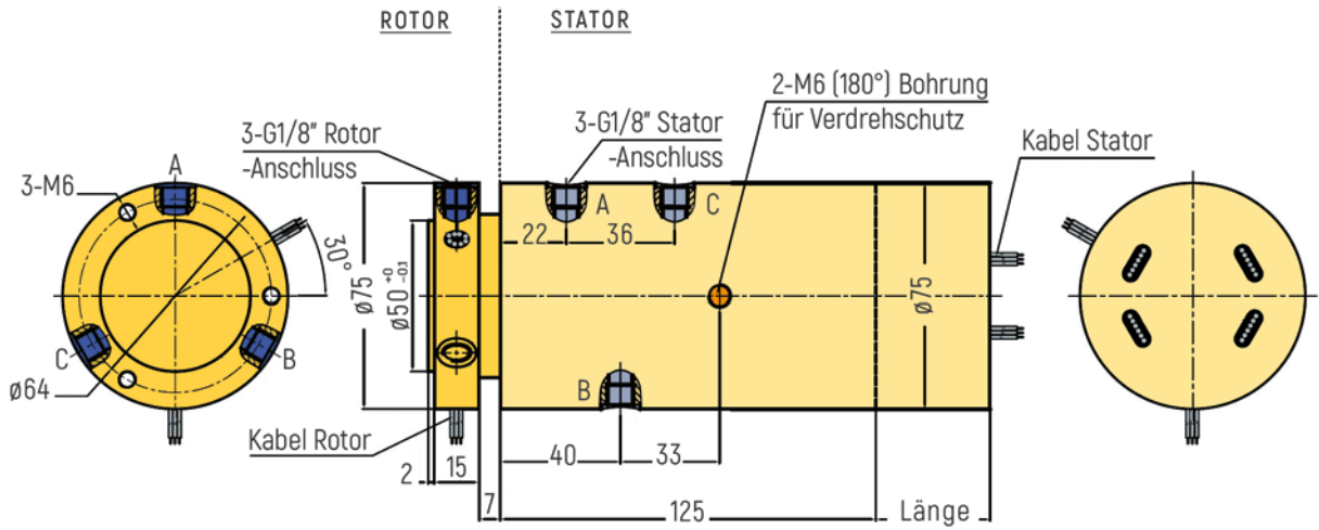
RX-PN1803-QS2-C - G1/8" Anschluss
