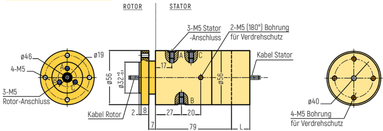
RX-PNM503-QS1-B - M5 Anschluss
