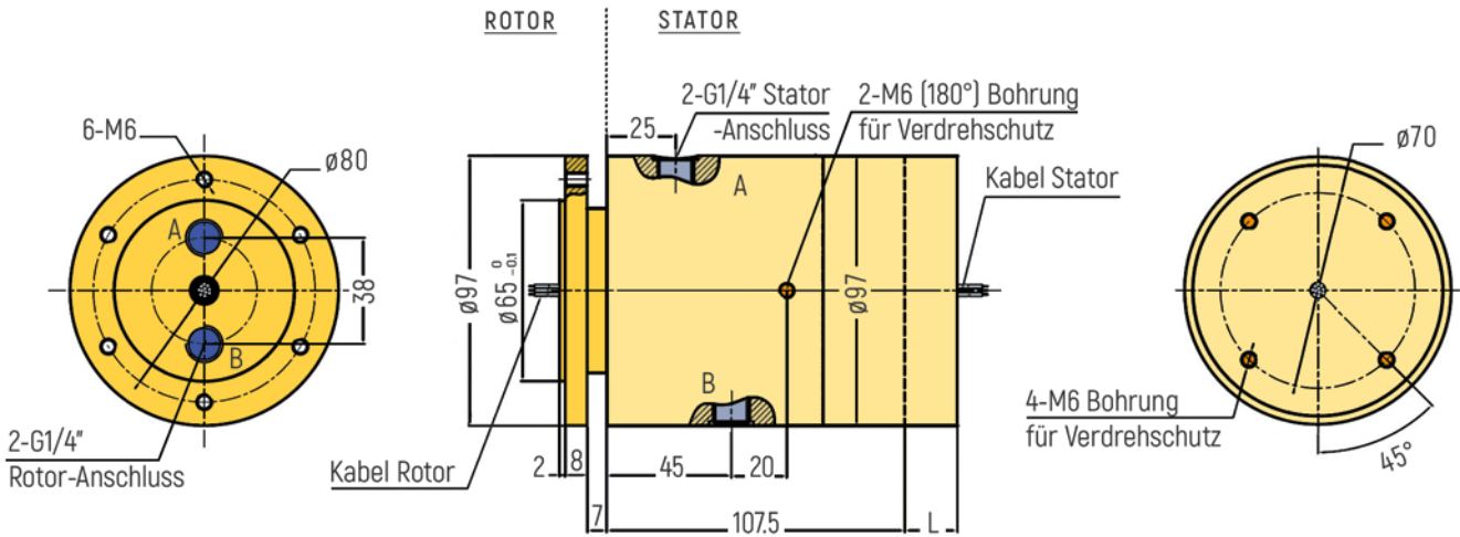
RX-PN1402-QS1-B - G1/4" Anschluss
