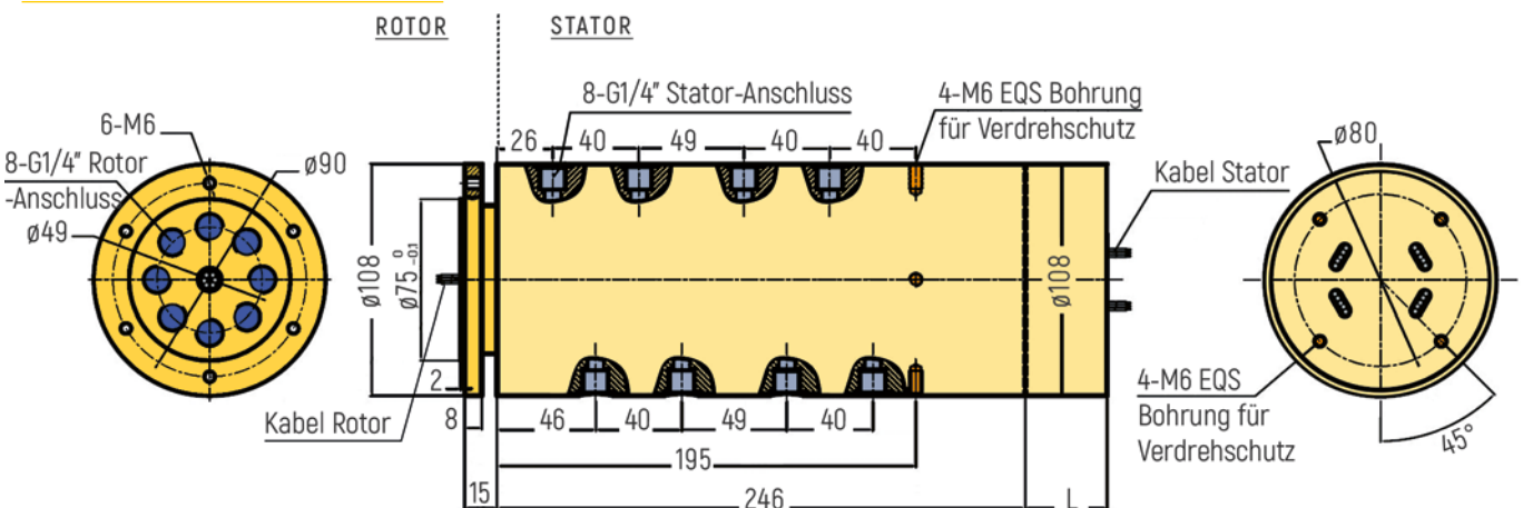
RX-PN1408-QS2-B - G1/4" Anschluss
