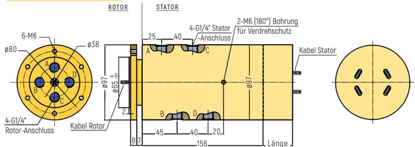
RX-PN1404-QS2-B - G1/4" Anschluss
