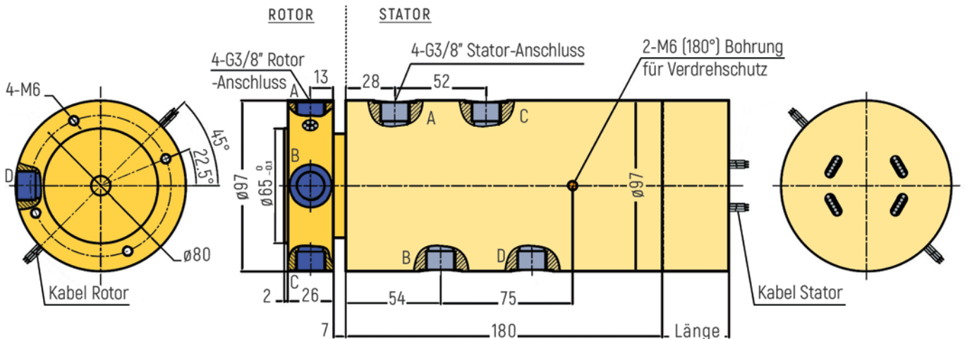
RX-PN3804-QS2-C - G3/8" Anschluss
