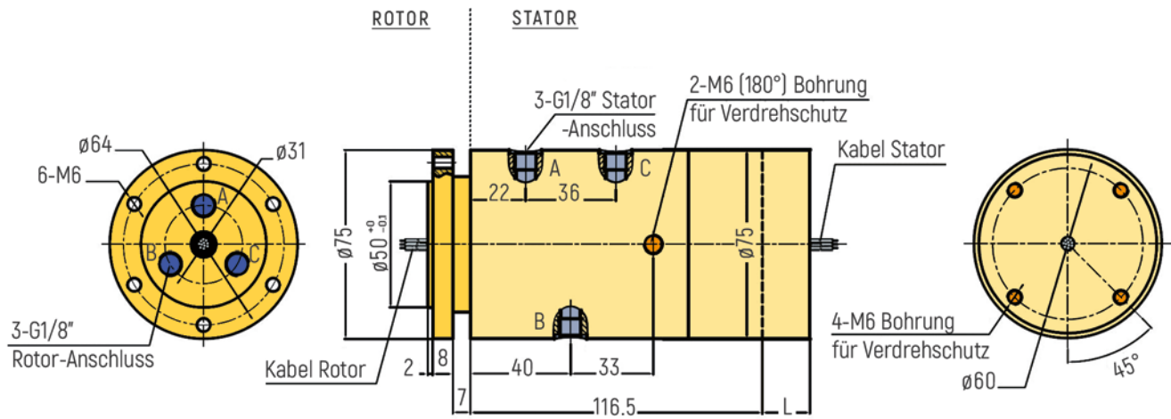
RX-PN1803-QS1-B - G1/8" Anschluss
