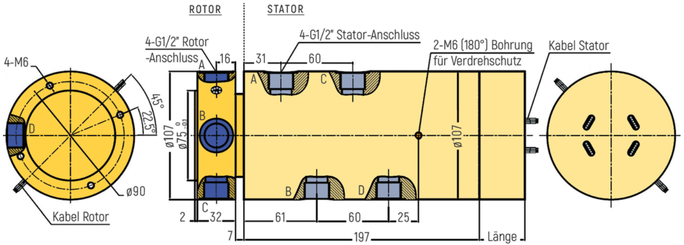
RX-PN1204-QS2-C - G1/2" Anschluss
