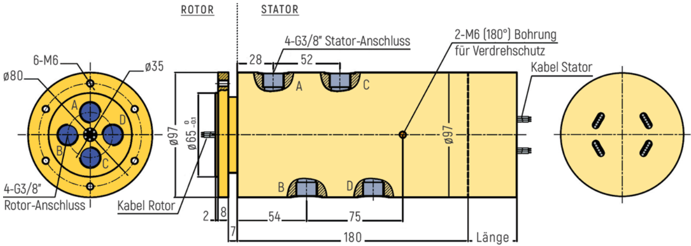
RX-PN3804-QS2-B - G3/8" Anschluss
