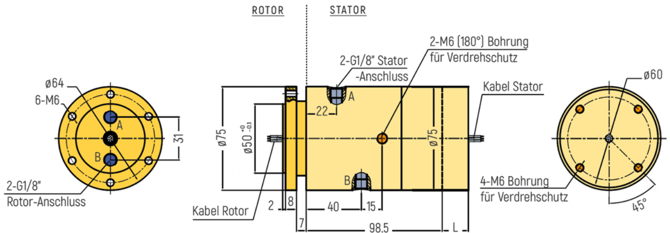
RX-PN1802-QS1-B - G1/8" Anschluss
