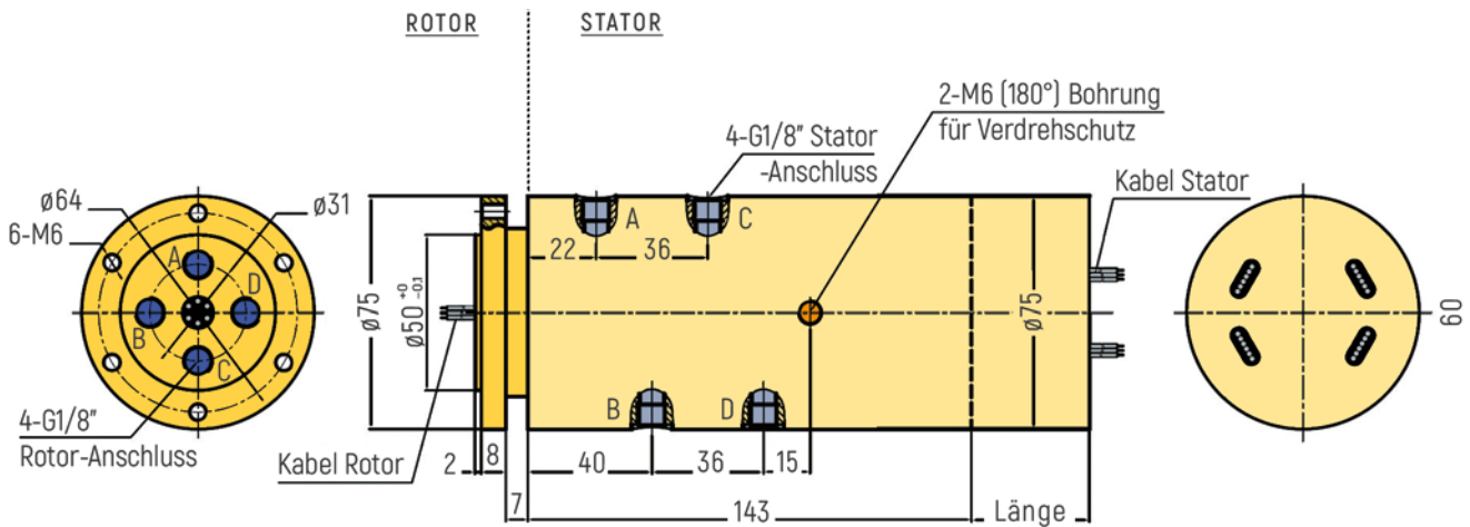
RX-PN1804-QS2-B - G1/8" Anschluss
