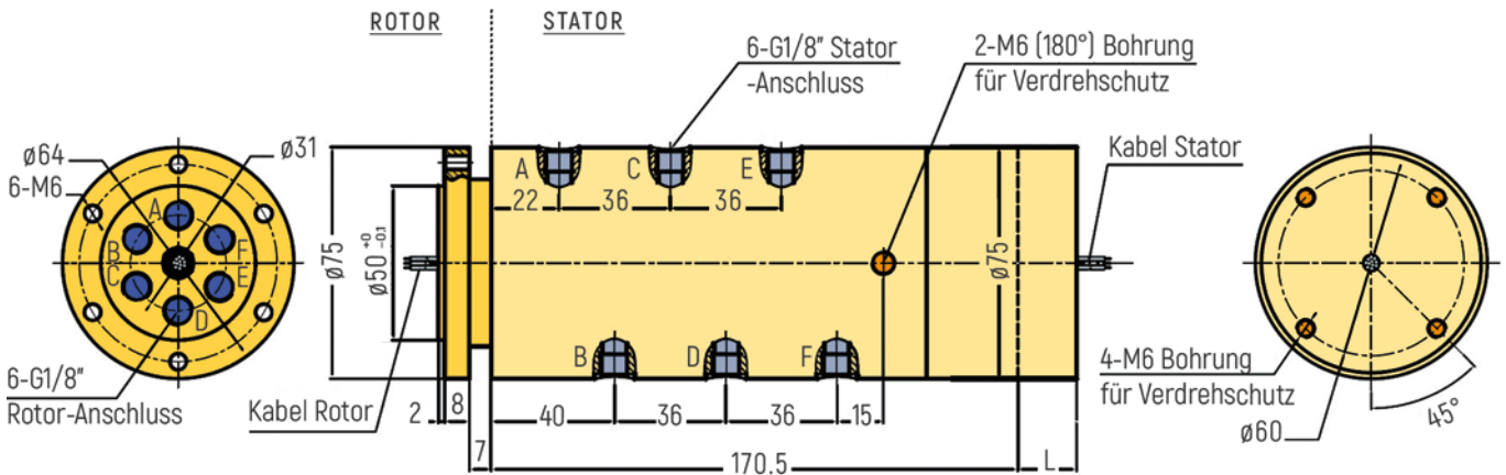
RX-PN1806-QS1-B - G1/8" Anschluss
