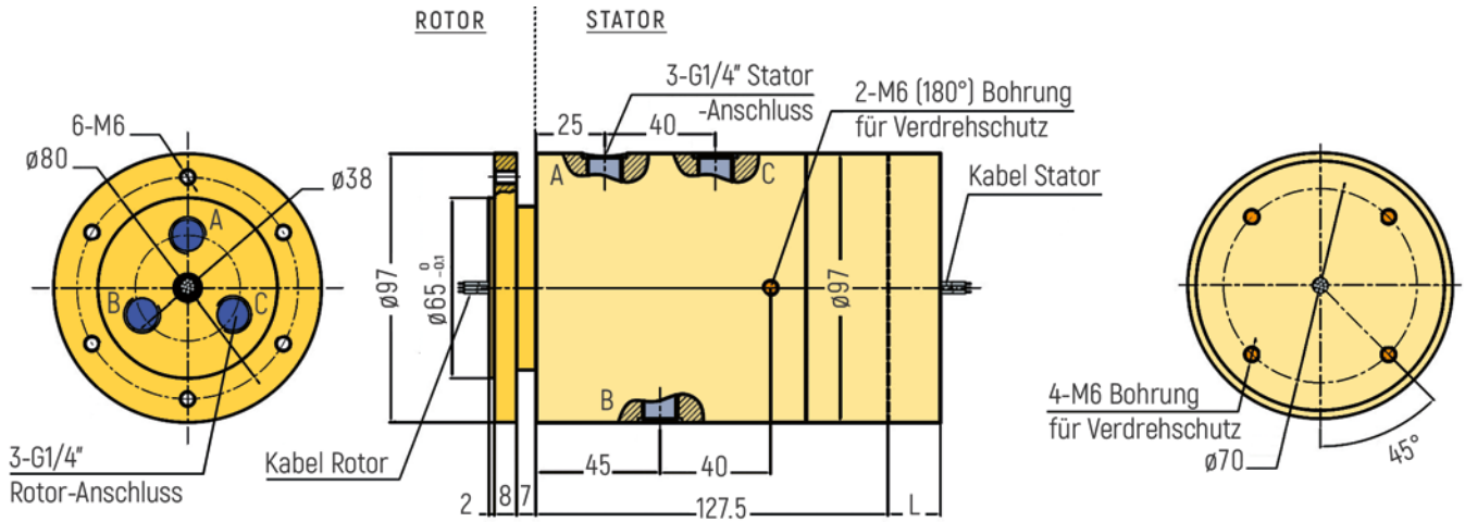
RX-PN1403-QS1-B - G1/4" Anschluss
