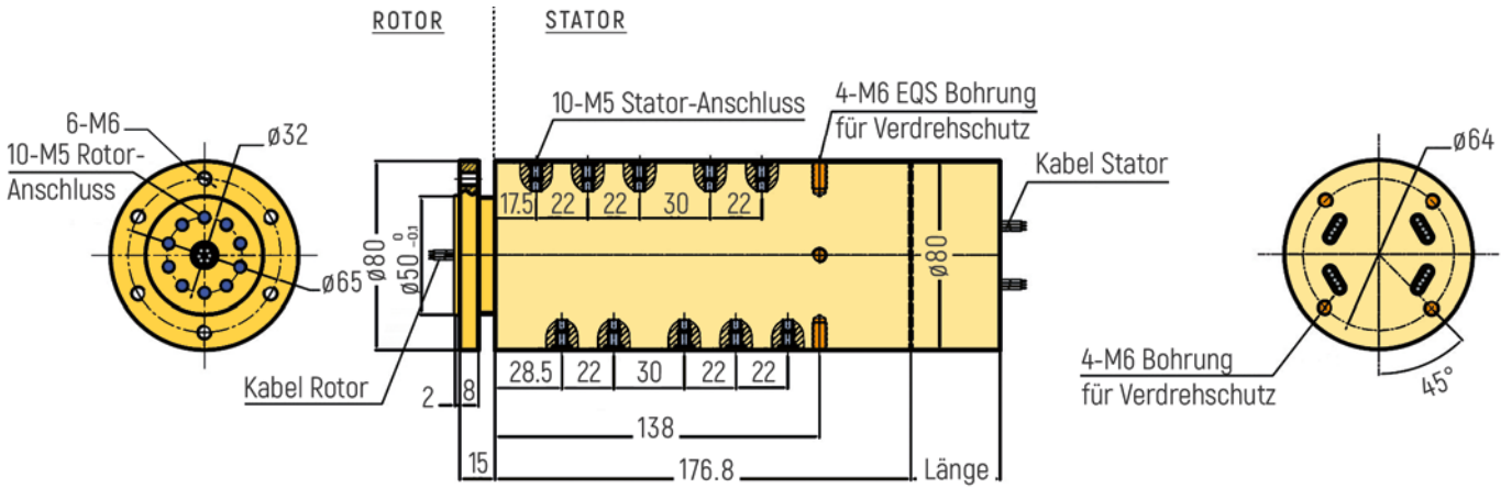
RX-PNM510-QS2-B - M5 Anschluss
