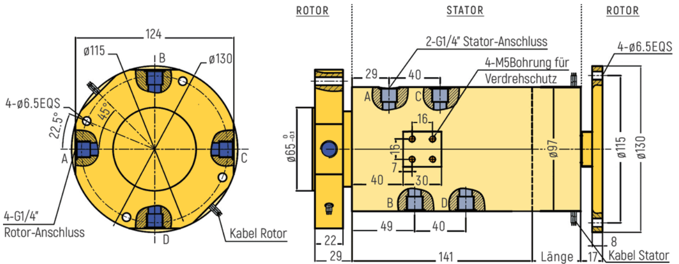
RX-PN1404-QS2-D - G1/4" Anschluss
