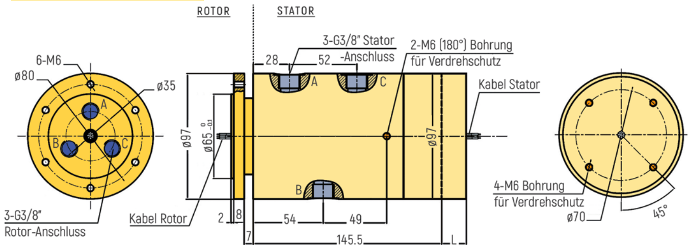
RX-PN3803-QS1-B - G3/8" Anschluss
