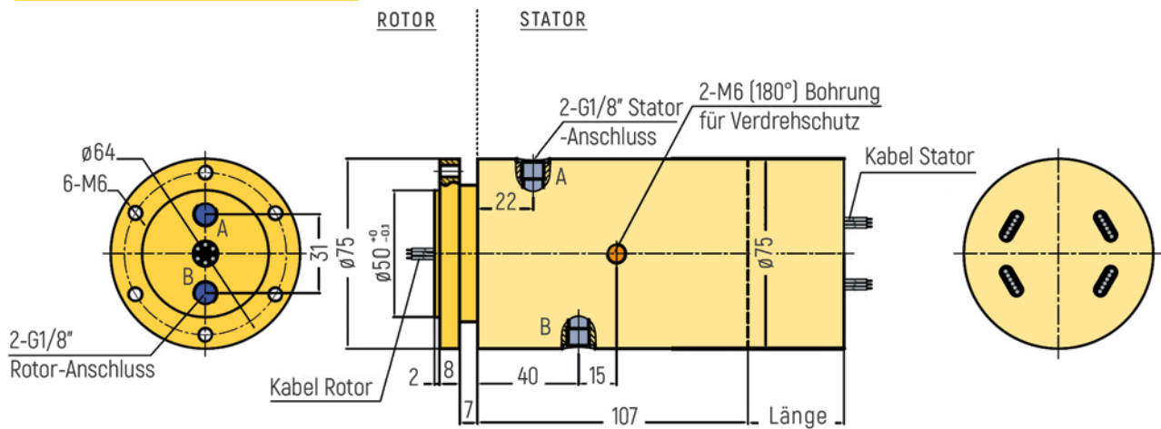
RX-PN1802-QS2-B - G1/8" Anschluss
