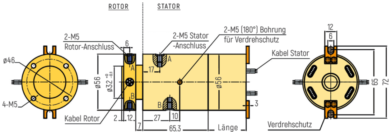
RX-PNM502-QS2-C - M5 Anschluss
