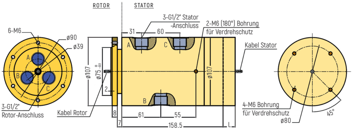
RX-PN1203-QS1-B - G1/2" Anschluss
