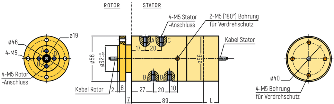
RX-PNM504-QS1-B - M5 Anschluss
