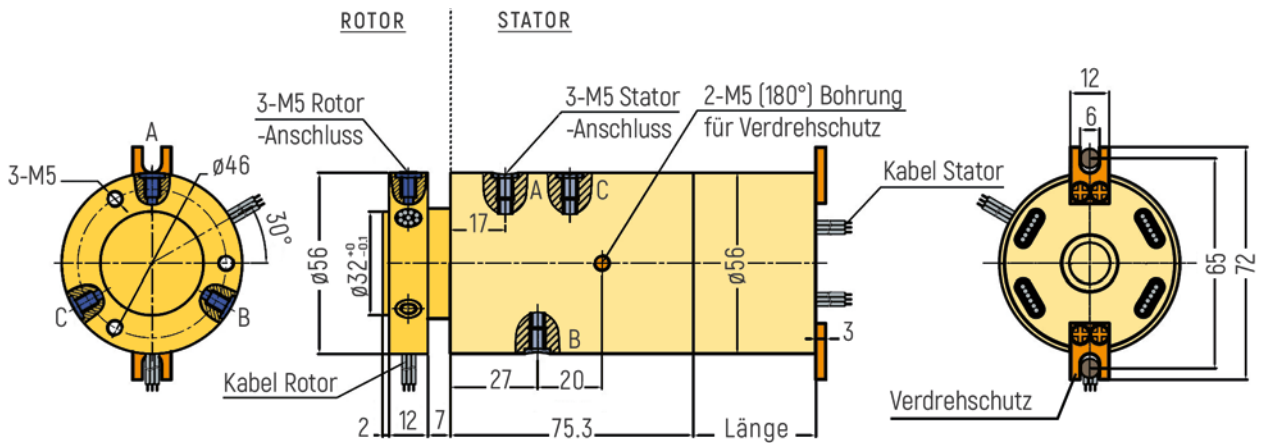
RX-PNM503-QS2-C - M5 Anschluss
