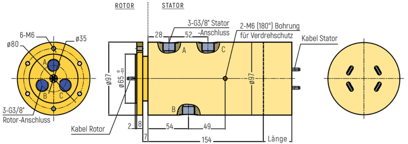
RX-PN3803-QS2-B - G3/8" Anschluss
