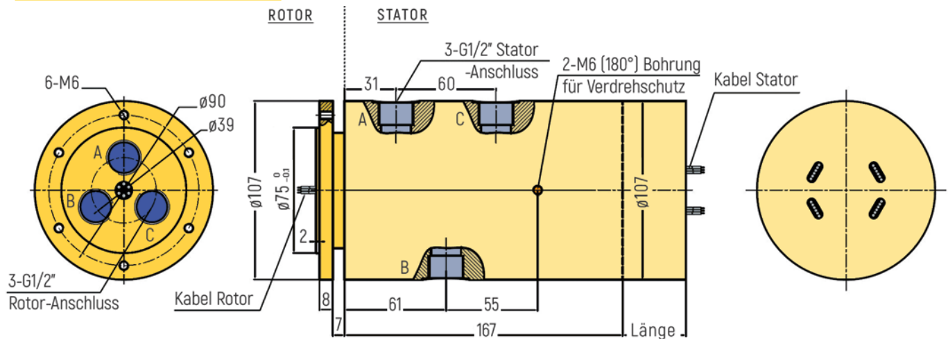
RX-PN1203-QS2-B - G1/2" Anschluss
