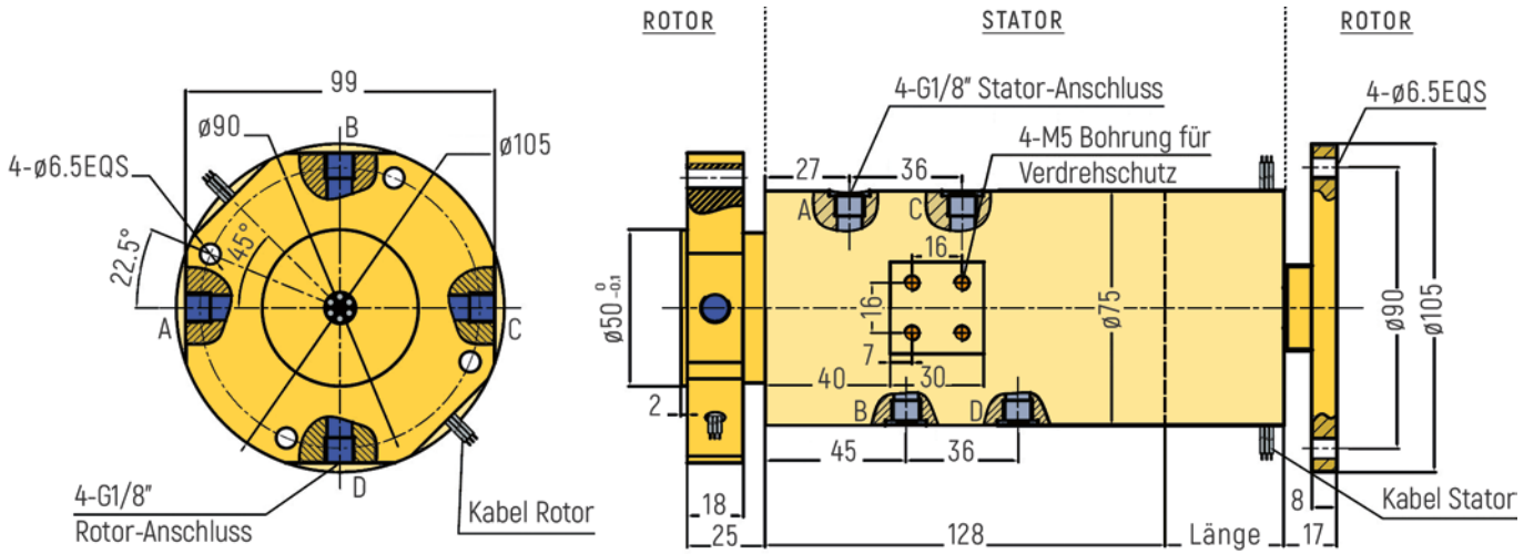
RX-PN1804-QS2-D - G1/8" Anschluss
