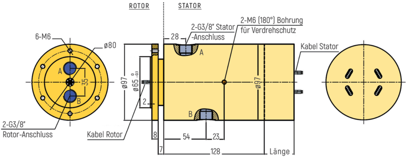
RX-PN3802-QS2-B - G3/8" Anschluss
