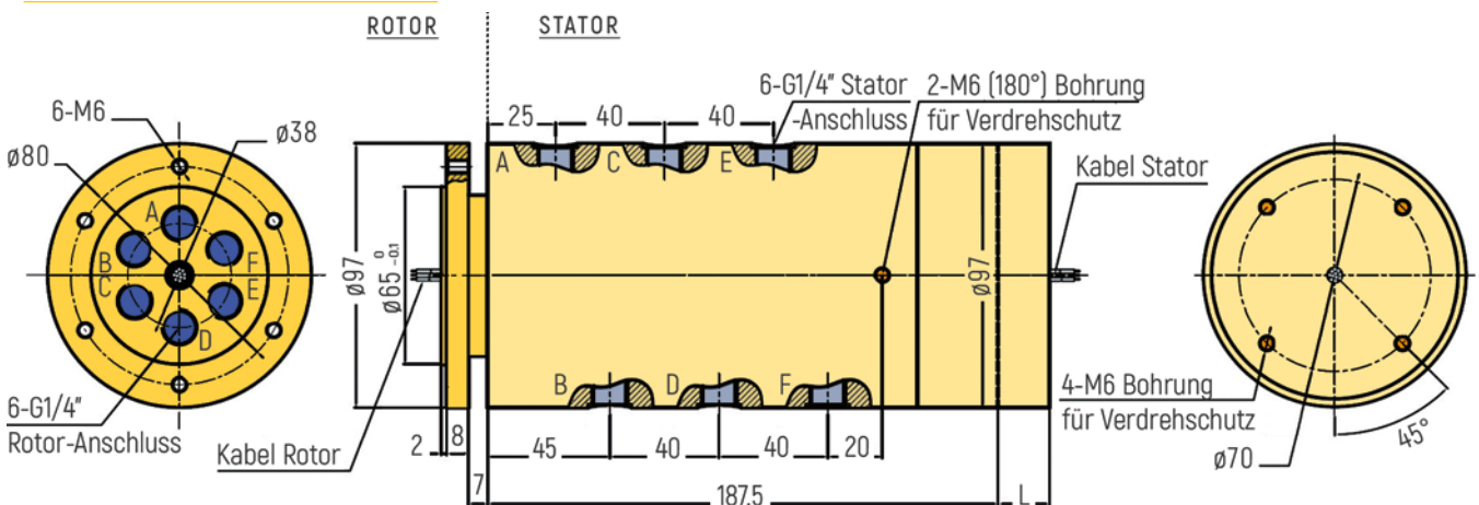
RX-PN1406-QS1-B - G1/4" Anschluss
