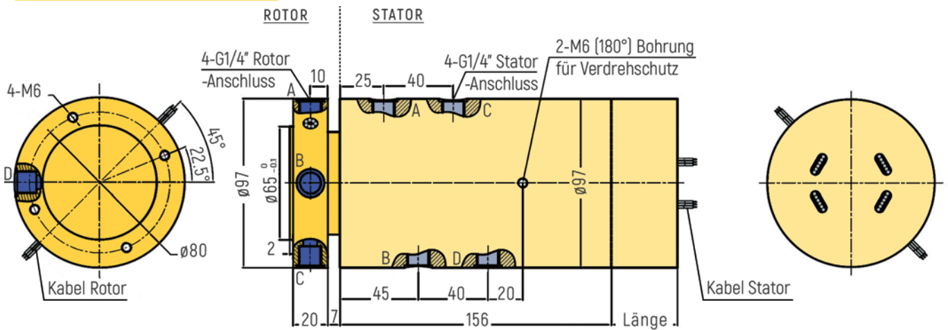
RX-PN1404-QS2-C - G1/4" Anschluss
