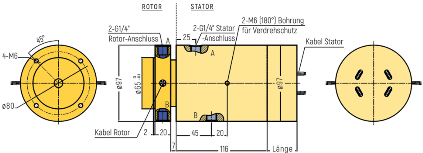
RX-PN1402-QS2-C - G1/4" Anschluss
