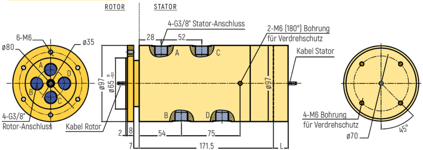
RX-PN3804-QS1-B - G3/8" Anschluss
