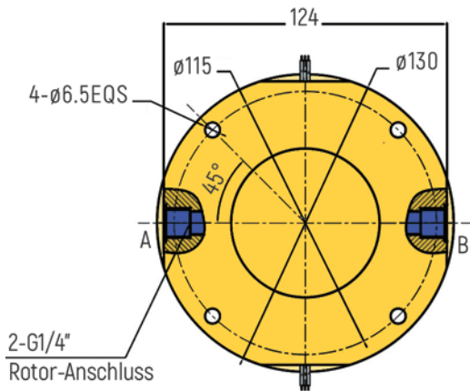
RX-PN1402-QS2-D - G1/4" Anschluss
