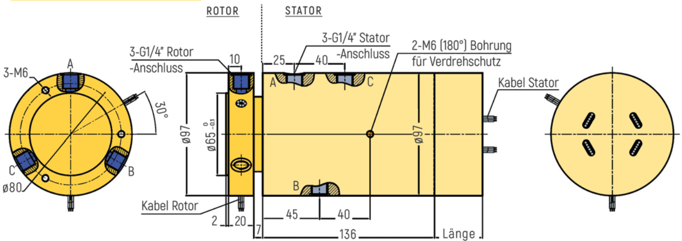
RX-PN1403-QS2-C - G1/4" Anschluss
