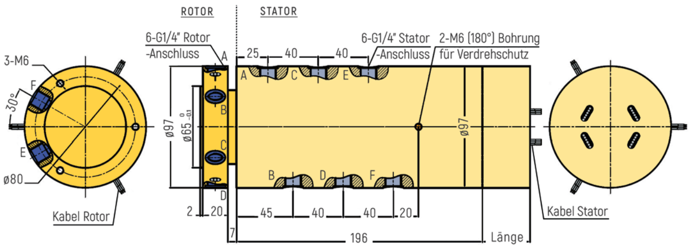
RX-PN1406-QS2-C - G1/4" Anschluss
