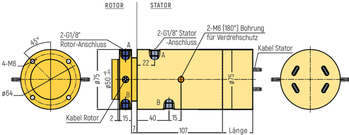
RX-PN1802-QS2-C - G1/8" Anschluss
