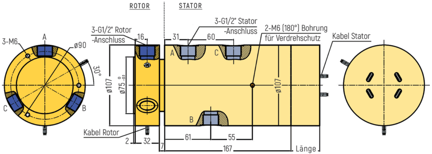
RX-PN1203-QS2-C - G1/2" Anschluss
