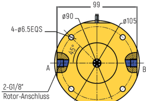
RX-PN1802-QS2-D - G1/8" Anschluss
