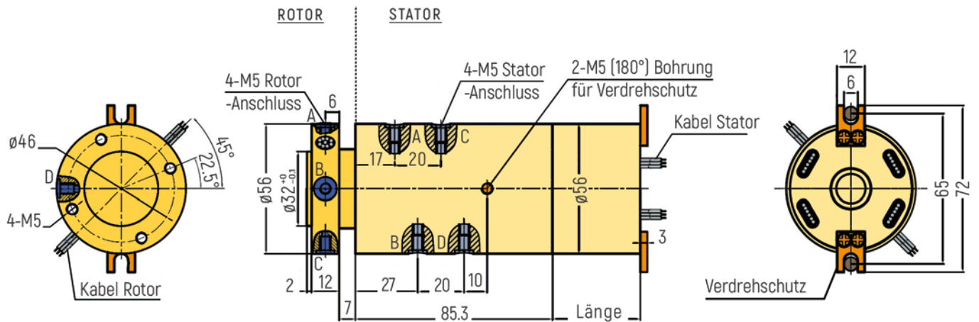
RX-PNM504-QS2-C - M5 Anschluss
