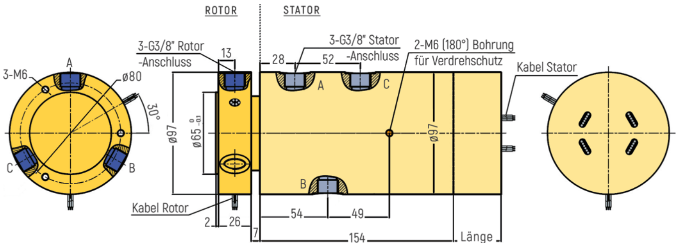
RX-PN3803-QS2-C - G3/8" Anschluss
