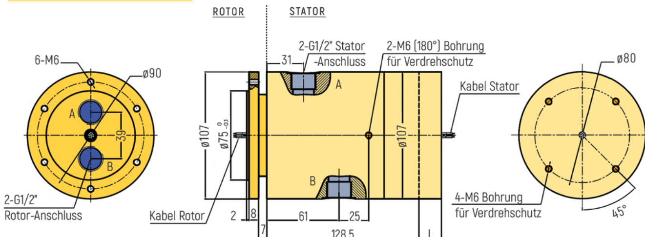
RX-PN1202-QS1-B - G1/2" Anschluss
