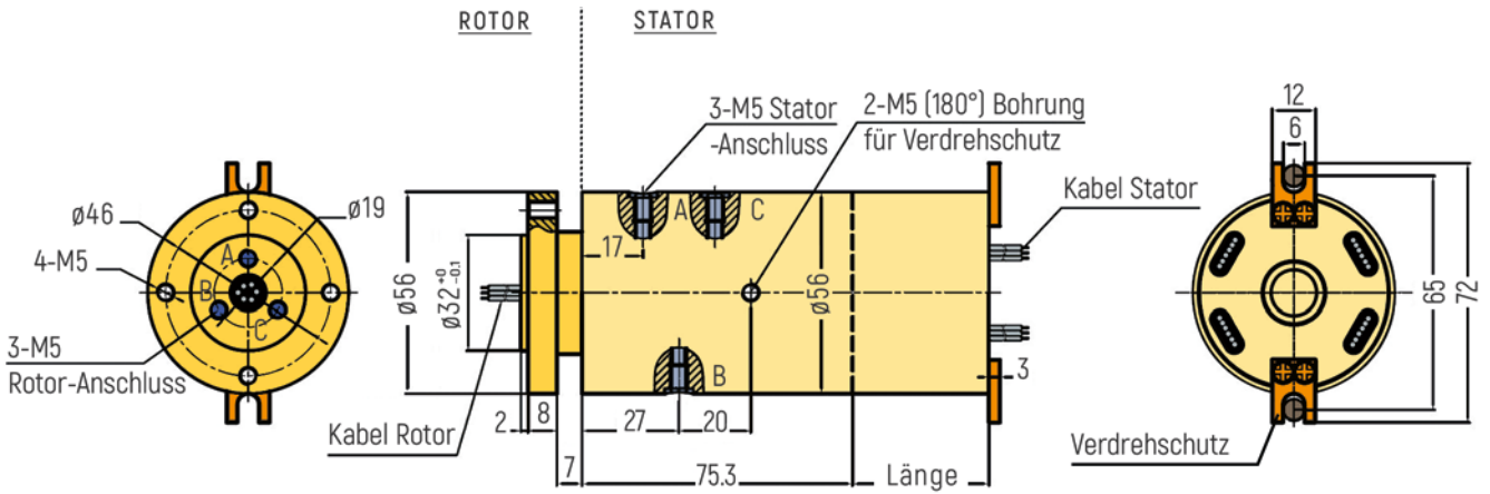
RX-PNM503-QS2-B - M5 Anschluss
