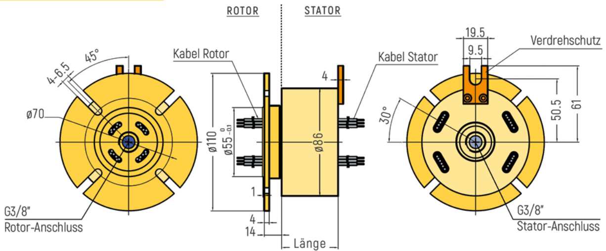
RX-PN3801-QS2-A - G3/8" Anschluss
