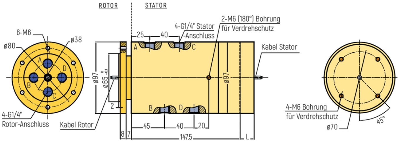
RX-PN1404-QS1-B - G1/4" Anschluss
