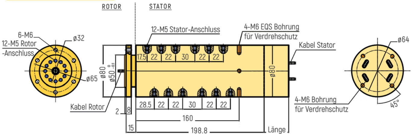
RX-PNM512-QS2-B - M5 Anschluss
