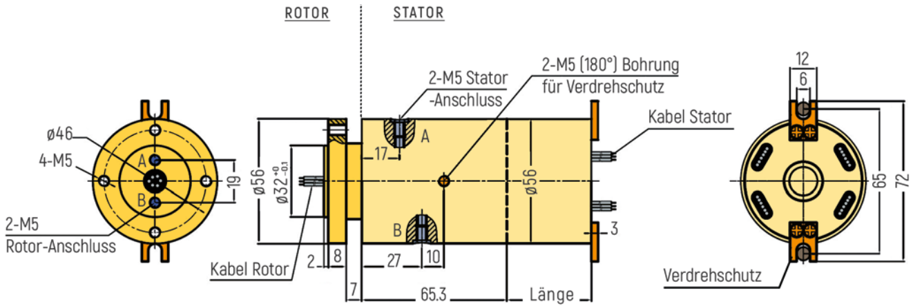
RX-PNM502-QS2-B - M5 Anschluss
