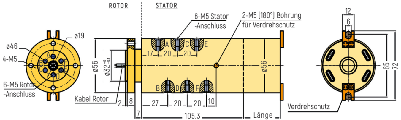
RX-PNM506-QS2-B - M5 Anschluss
