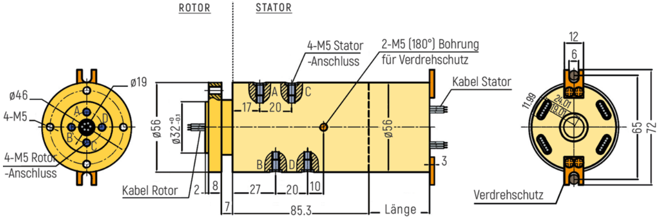
RX-PNM504-QS2-B - M5 Anschluss
