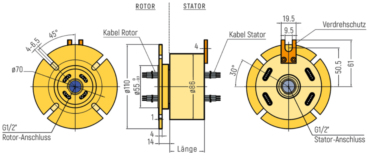
RX-PN1201-QS2-A - G1/2" Anschluss
