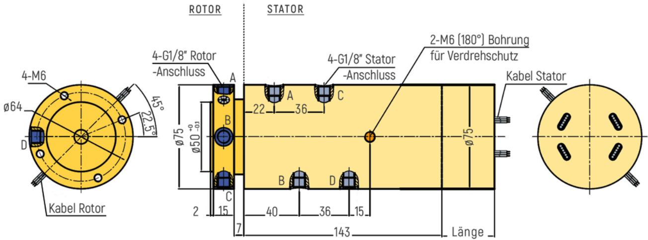
RX-PN1804-QS2-C - G1/8" Anschluss
