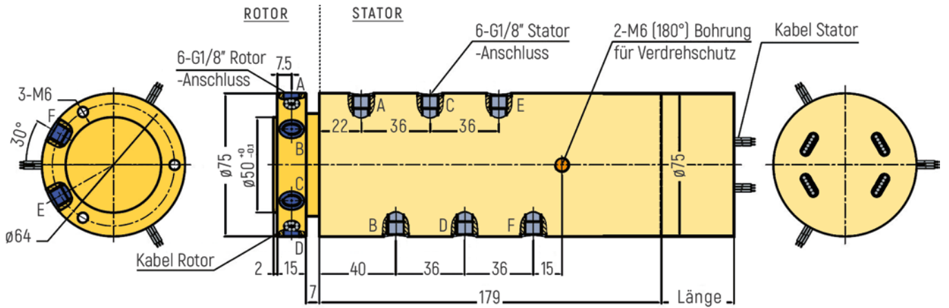
RX-PN1806-QS2-C - G1/8" Anschluss
