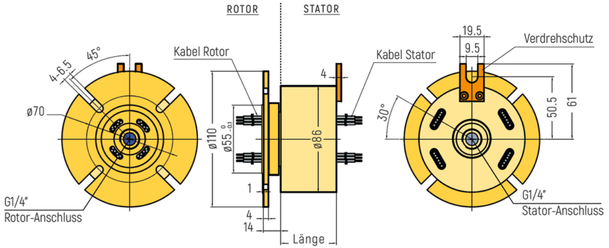
RX-PN1401-QS2-A - G1/4" Anschluss
