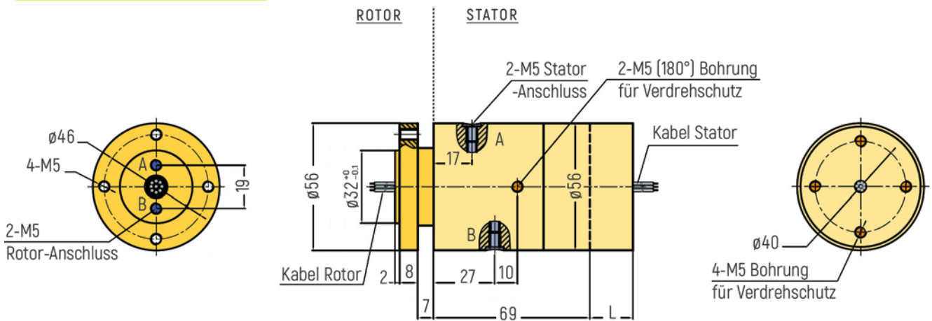
RX-PNM502-QS1-B - M5 Anschluss
