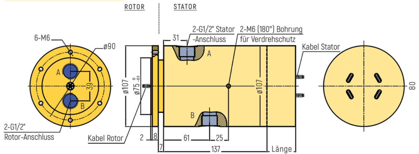
RX-PN1202-QS2-B - G1/2" Anschluss
