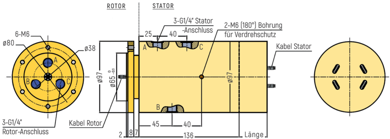
RX-PN1403-QS2-B - G1/4" Anschluss
