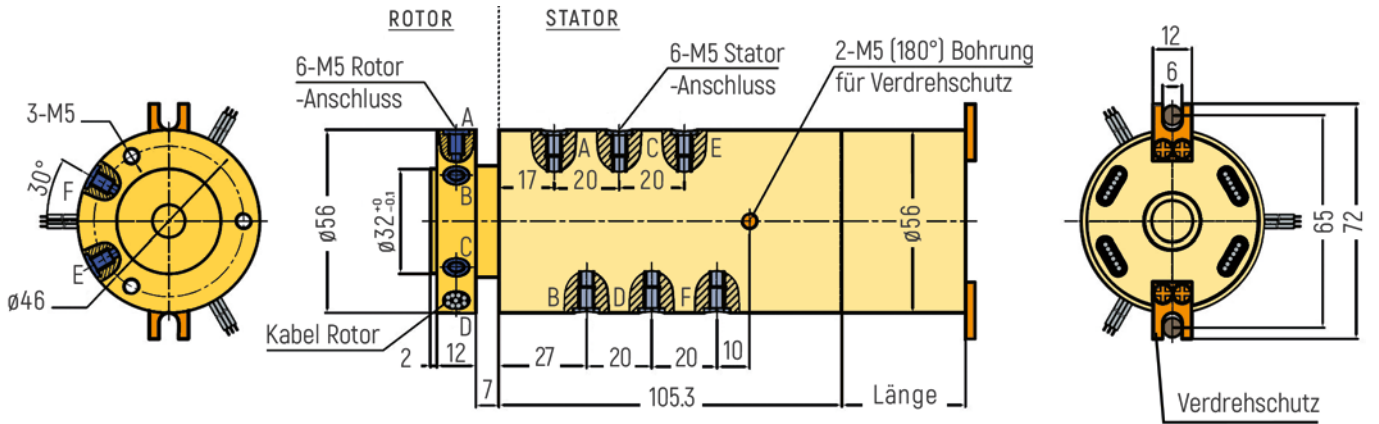
RX-PNM506-QS2-C - M5 Anschluss
