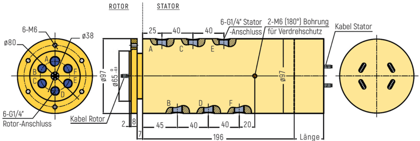
RX-PN1406-QS2-B - G1/4" Anschluss
