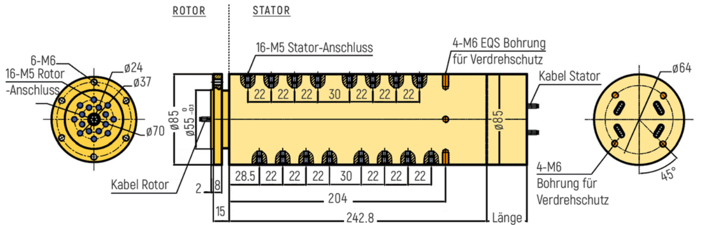
RX-PNM516-QS2-B - M5 Anschluss
