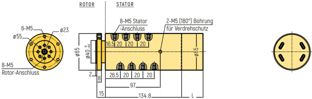
RX-PNM508-QS2-B - M5 Anschluss
