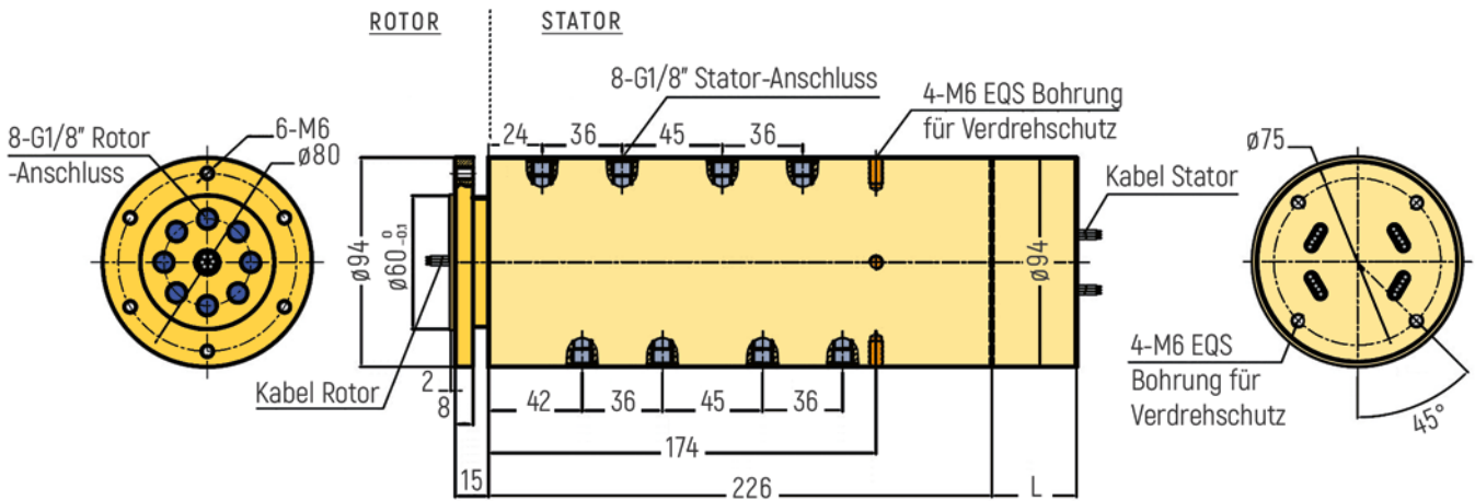
RX-PN1808-QS2-B - G1/8" Anschluss
