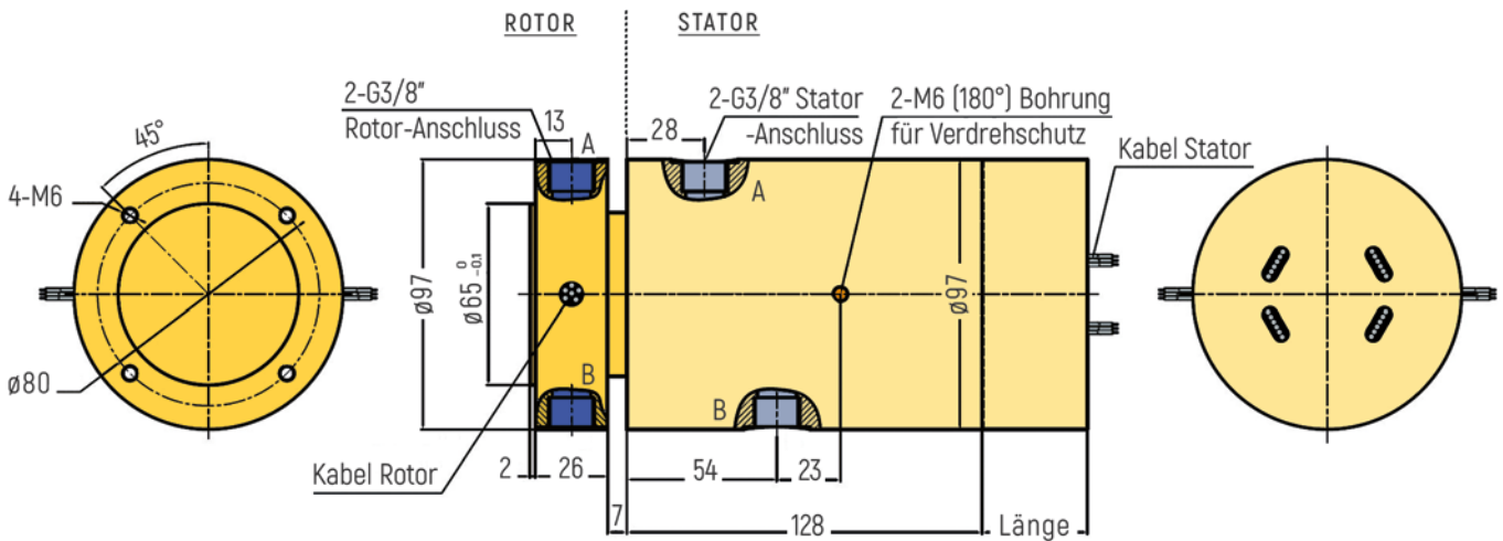
RX-PN3802-QS2-C - G3/8" Anschluss
