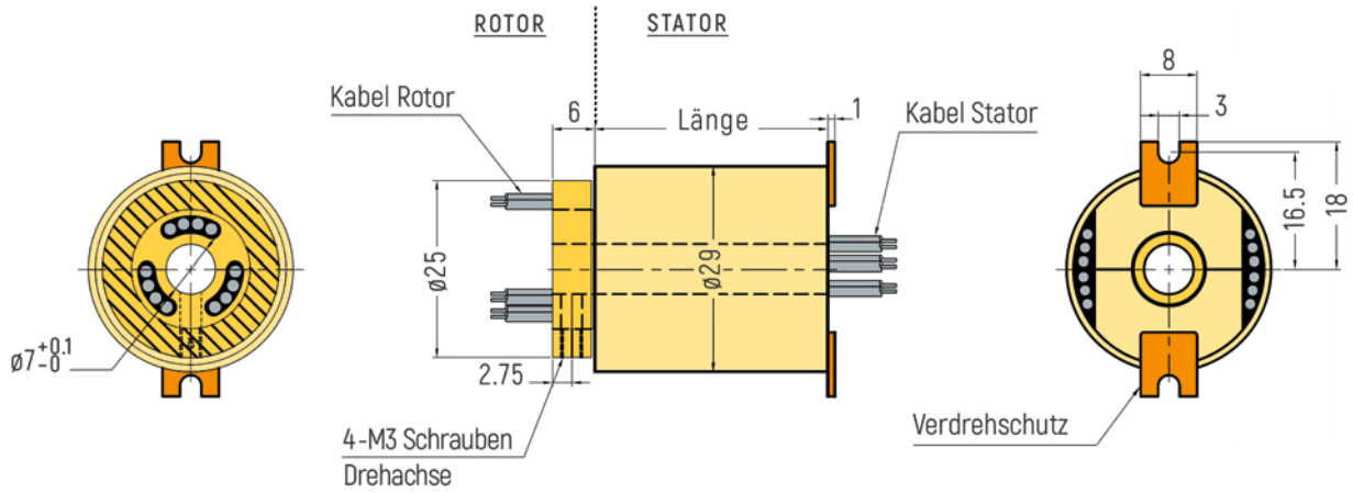
RX-HS007B - Durchmesser Hohlwelle 7mm
