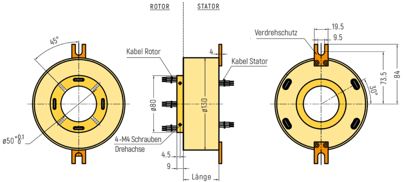
RX-HS050B - Durchmesser Hohlwelle 50mm
