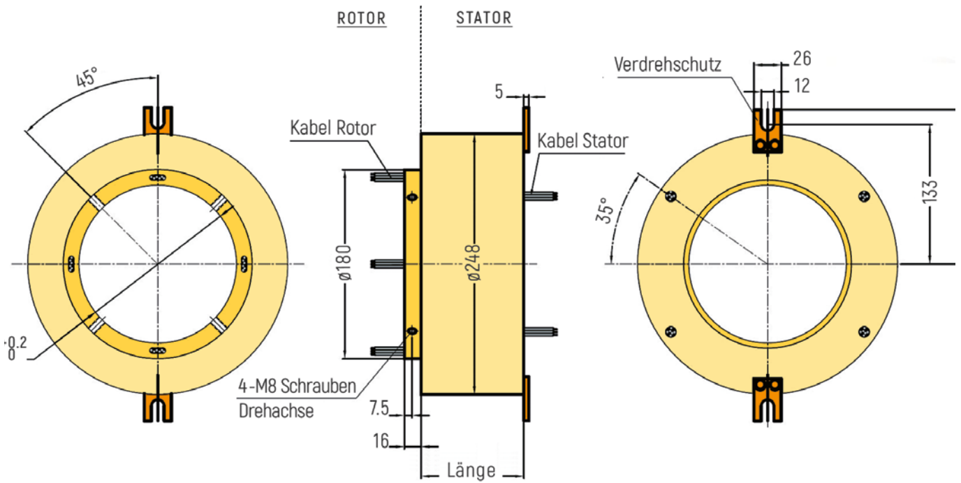
RX-HS150A - Durchmesser Hohlwelle 150mm
