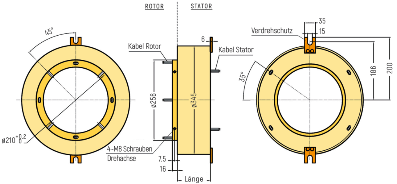
RX-HS210A - Durchmesser Hohlwelle 210mm
