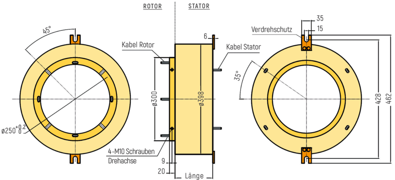
RX-HS250A - Durchmesser Hohlwelle 250mm
