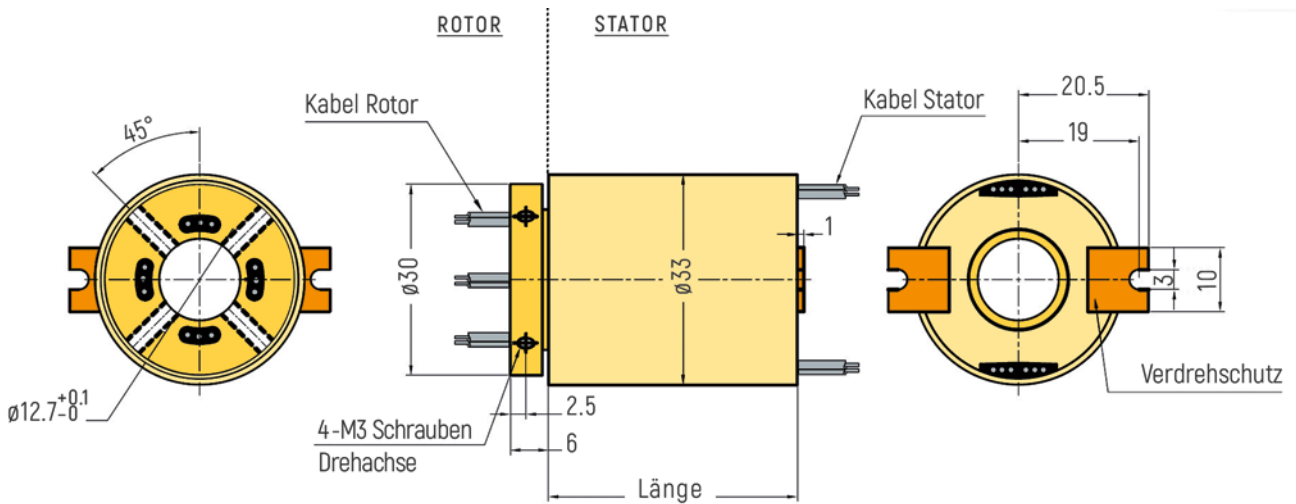
RX-HS012A - Durchmesser Hohlwelle 12,7mm
