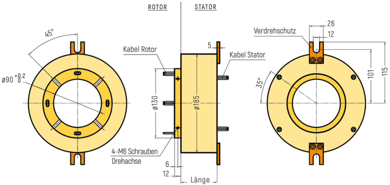
RX-HS090A - Durchmesser Hohlwelle 90mm
