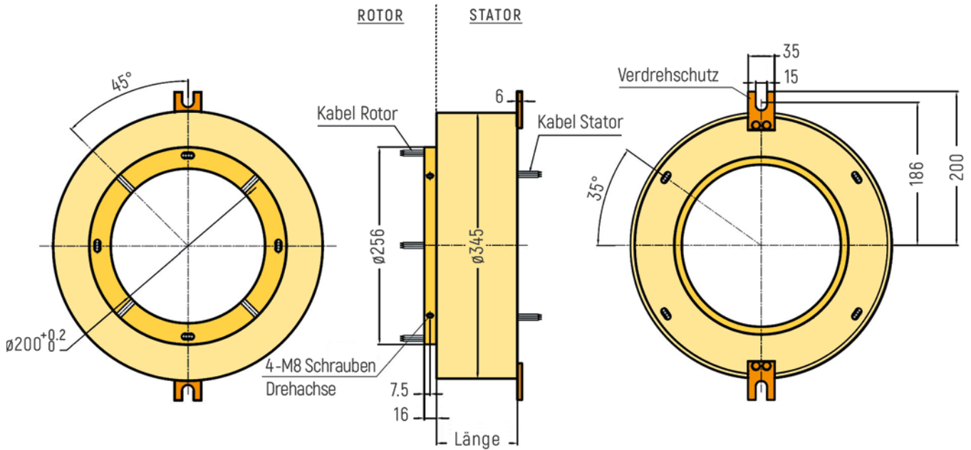
RX-HS200A - Durchmesser Hohlwelle 200mm
