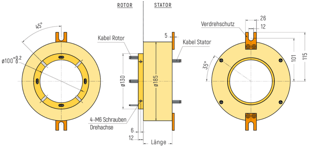
RX-HS100A - Durchmesser Hohlwelle 100mm
