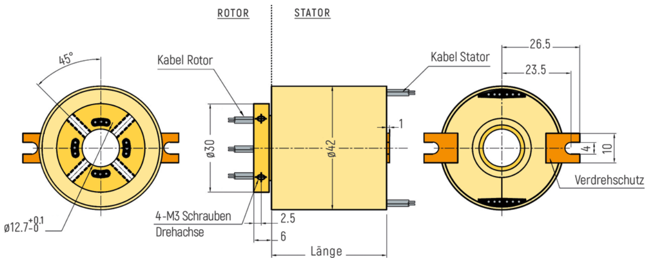
RX-HS012B - Durchmesser Hohlwelle 12,7mm
