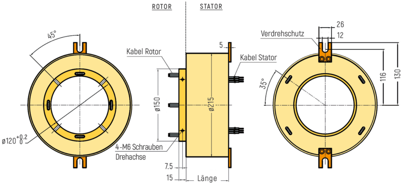
RX-HS120A - Durchmesser Hohlwelle 120mm
