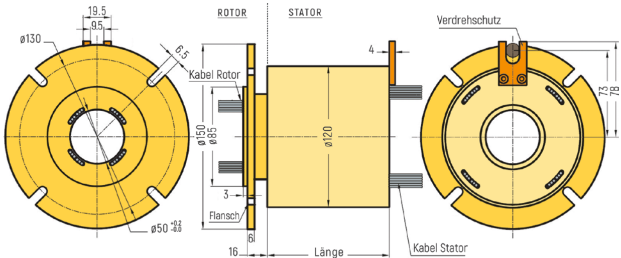
RX-ETH502 - Optionale Flanschversion (Zeichnung nur beispielhaft, weitere Details auf Anfrage)
