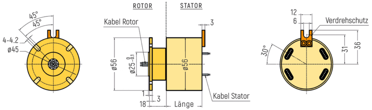
RX-RF056A - Schleifring mit Rotor-Flansch
