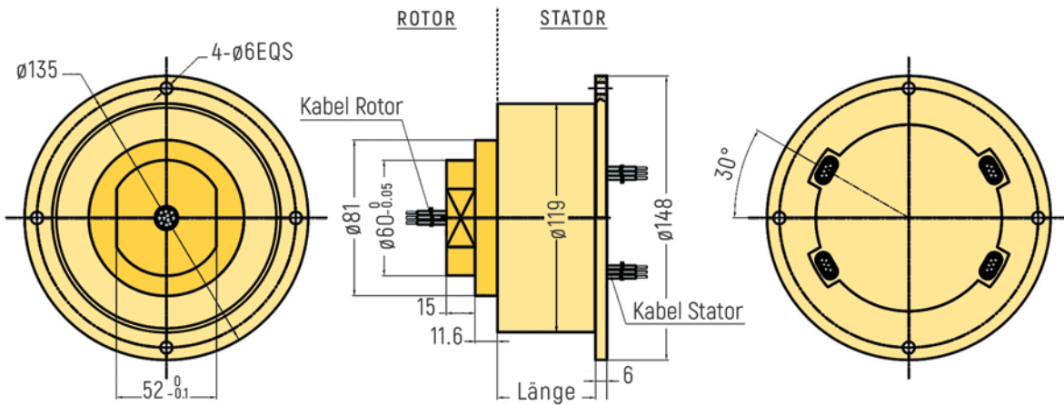
RX-SF119B - Schleifring mit Stator-Flansch
