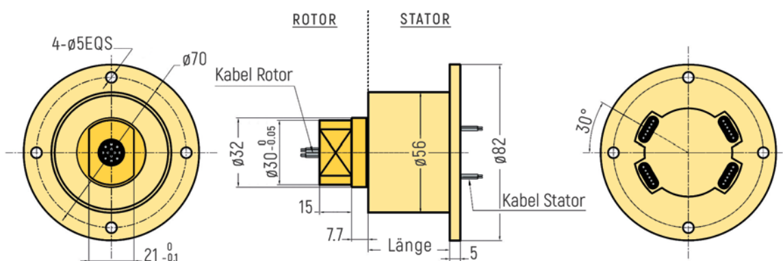
RX-SF056B - Schleifring mit Stator-Flansch
