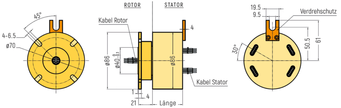
RX-RF086A - Schleifring mit Rotor-Flansch
