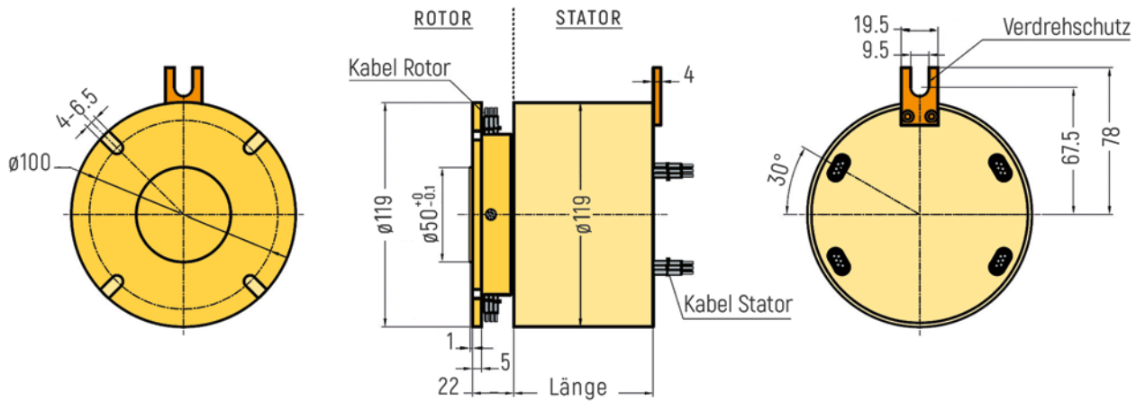
RX-RF119B - Schleifring mit Rotor-Flansch
