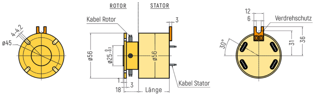
RX-RF056B - Schleifring mit Rotor-Flansch
