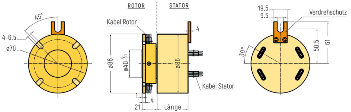
RX-RF086B - Schleifring mit Rotor-Flansch
