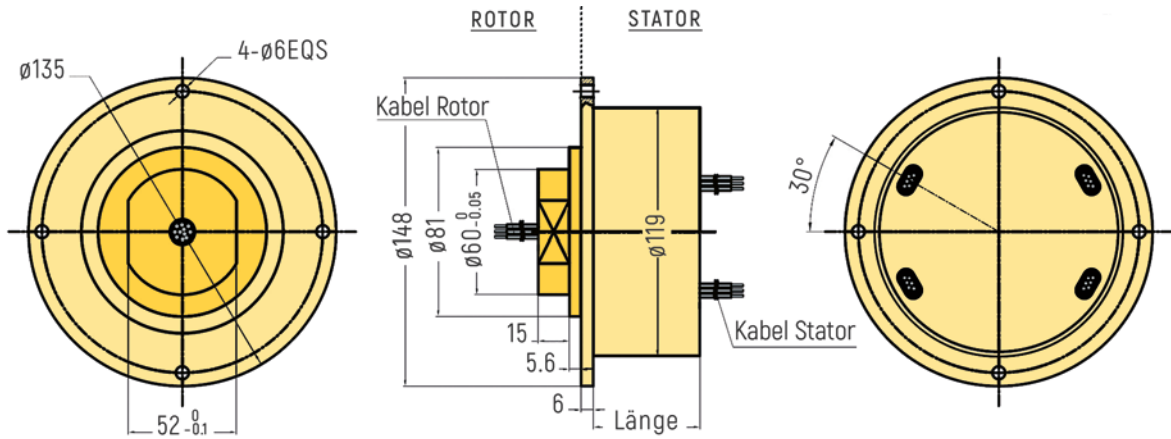
RX-SF119A - Schleifring mit Stator-Flansch
