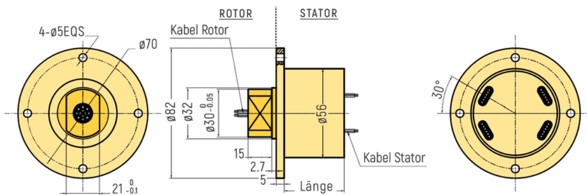
RX-SF056A - Schleifring mit Stator-Flansch
