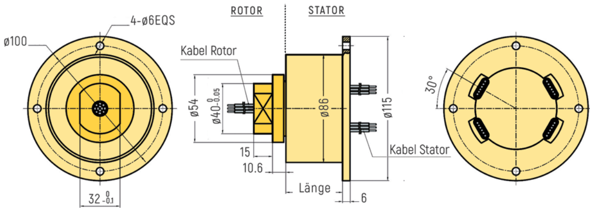
RX-SF086B - Schleifring mit Stator-Flansch
