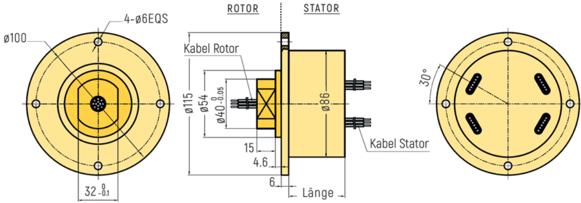
RX-SF086A - Schleifring mit Stator-Flansch
