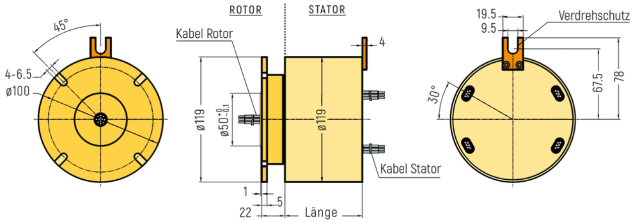
RX-RF119A - Schleifring mit Rotor-Flansch
